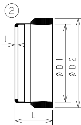
TM-Ⅱパッキン寸法表
