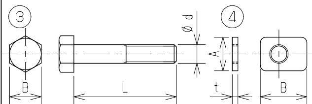
六角ボルト・LKナット寸法表
