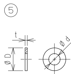
平座金寸法表
