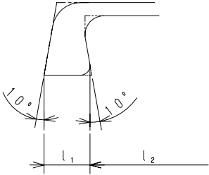
呼び32・250の形状
